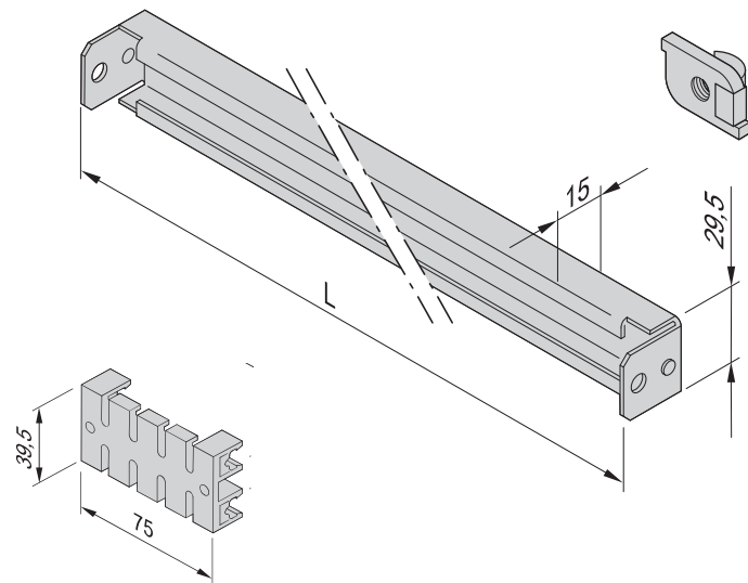
01006071 Kabelabfangeleiste
