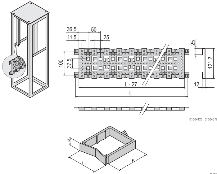
Kabelöse
