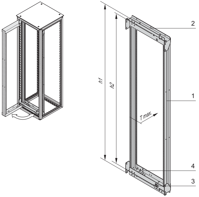
01005055 Schwenkrahmenarretierung
